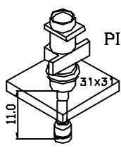
AQNA-3249 PICK-UP NOZZLE \phi 20.0 (OD= \phi 20.0 ) FUJI , IP3
