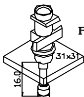
AQNA-3118 PICK-UP NOZZLE \phi 0.7 (OD= \phi 0.7 ) FUJI , IP3
