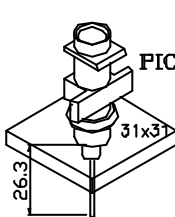
AQNA-3332 PICK-UP NOZZLE \phi 6.5 (OD= \phi 6.5 ) FUJI , IP3
