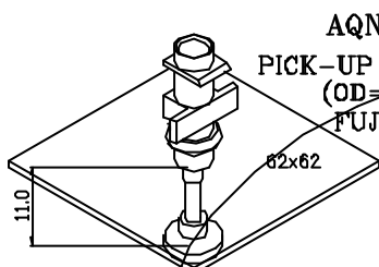
AQNA-3302 PICK-UP NOZZLE \phi 7.0 (OD= \phi 7.0 ) FUJI , IP3
