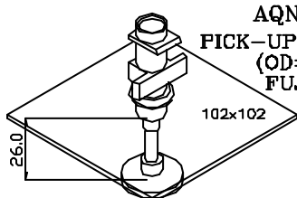
AQNA-3249 PICK-UP NOZZLE \phi 20.0 (OD= \phi 20.0 ) FUJI , IP3
