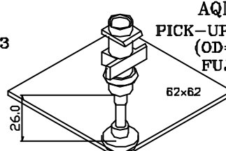
AQNA-3238 PICK-UP NOZZLE \phi 15.0 (OD= \phi 15.0 ) FUJI , IP3
