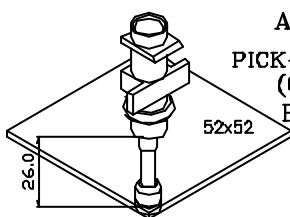
AQNA-3209 PICK-UP NOZZLE \phi 20.0 (OD= \phi 20.0 ) FUJI , IP3
