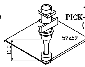
AQNA-3258 PICK-UP NOZZLE \phi 7.0 (OD= \phi 7.0 ) FUJI , IP3
