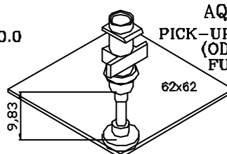
AQNA-3268 PICK-UP NOZZLE \phi 10.0 (OD= \phi 10.0 ) FUJI , IP3
