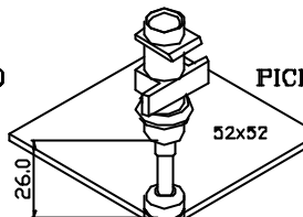
AQNA-3178 PICK-UP NOZZLE \phi 7.0 (OD= \phi 7.0 ) FUJI , IP3
